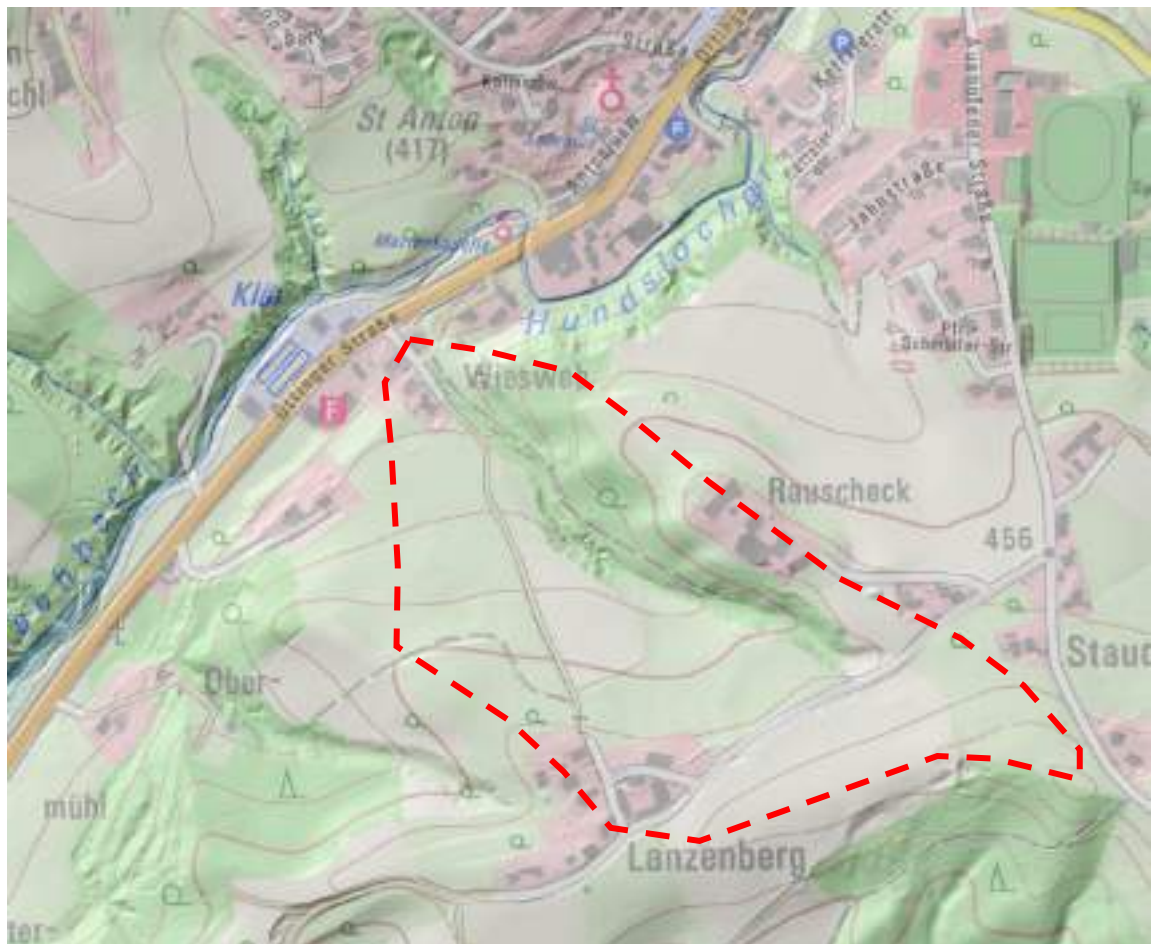
Abbildung 27: Einzugsgebiet Öttinger Straße / Wiesweb
