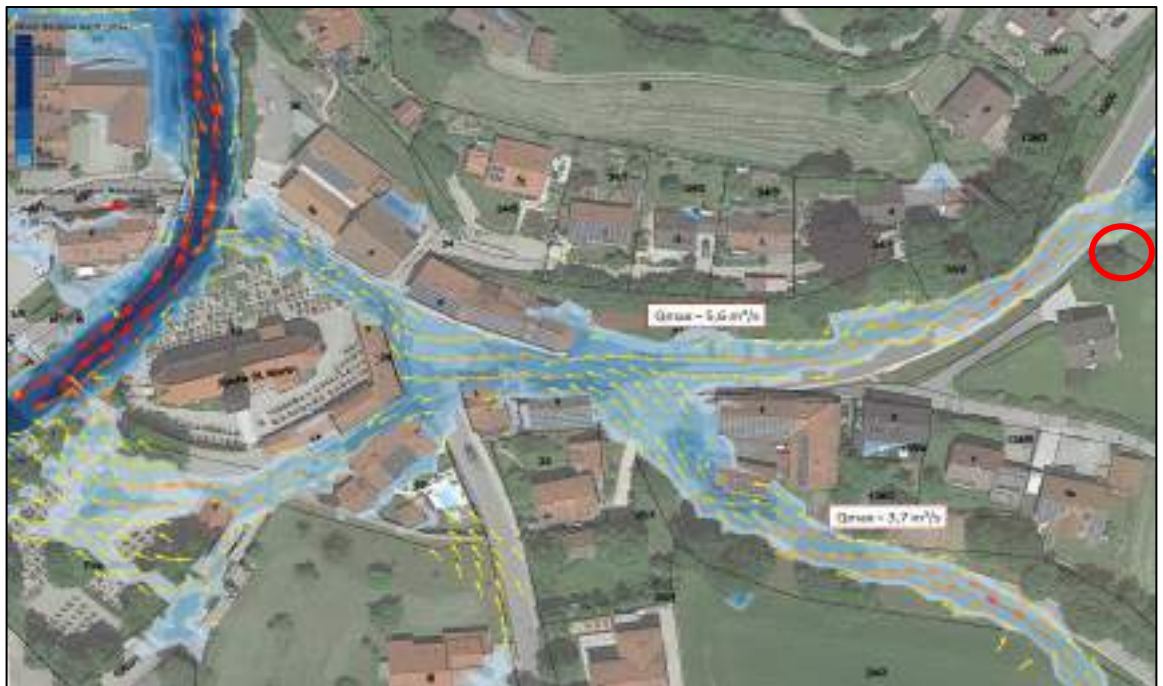
Abbildung 22: N100 Ereignis mit Fließgeschwindigkeiten in Reischach-Ost
