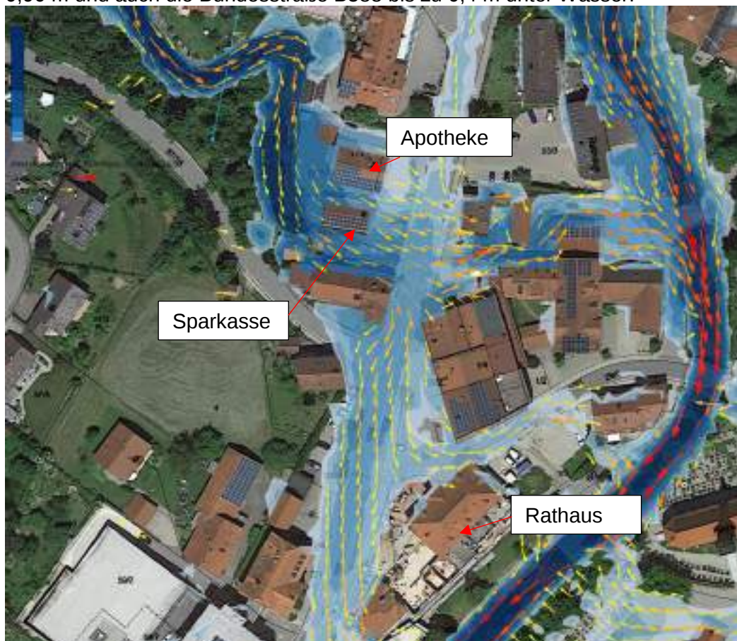
Abbildung 26: N100 Ereignis mit Fließgeschwindigkeiten im Ortskern Reischach
