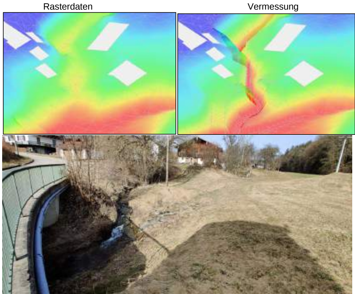
Abbildung 10: Vergleich Modellgüte am Josef-Straubinger-Weg
