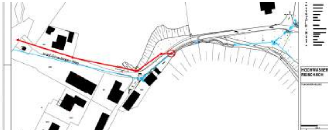
Abbildung 40: Neubau/Ertüchtigung RW-Kanal Josef-Straubinger-Weg
