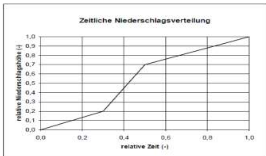
Abbildung 7: Zeitliche Niederschlagsverteilung nach DVWK
