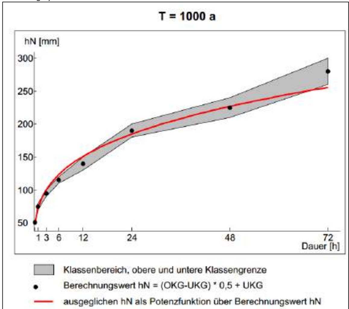
Abbildung 4: Potenzfunktion zur Ermittlung der Niederschlagswerte für N1000
