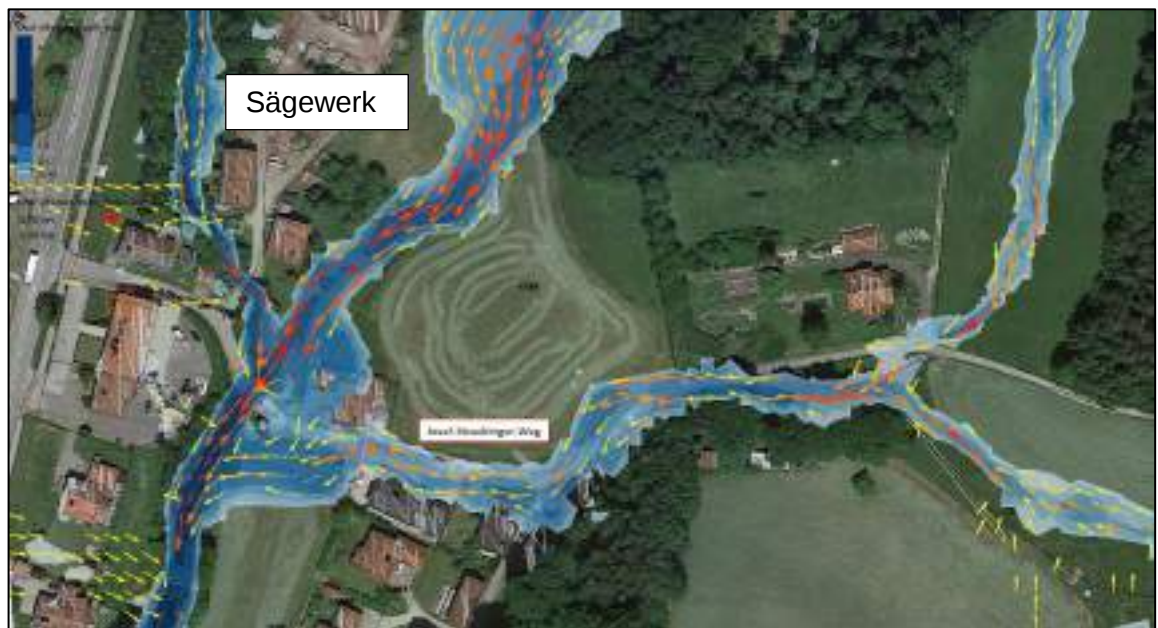
Abbildung 18: N100 Ereignis mit Fließgeschwindigkeiten im Josef-Straubinger-Weg
